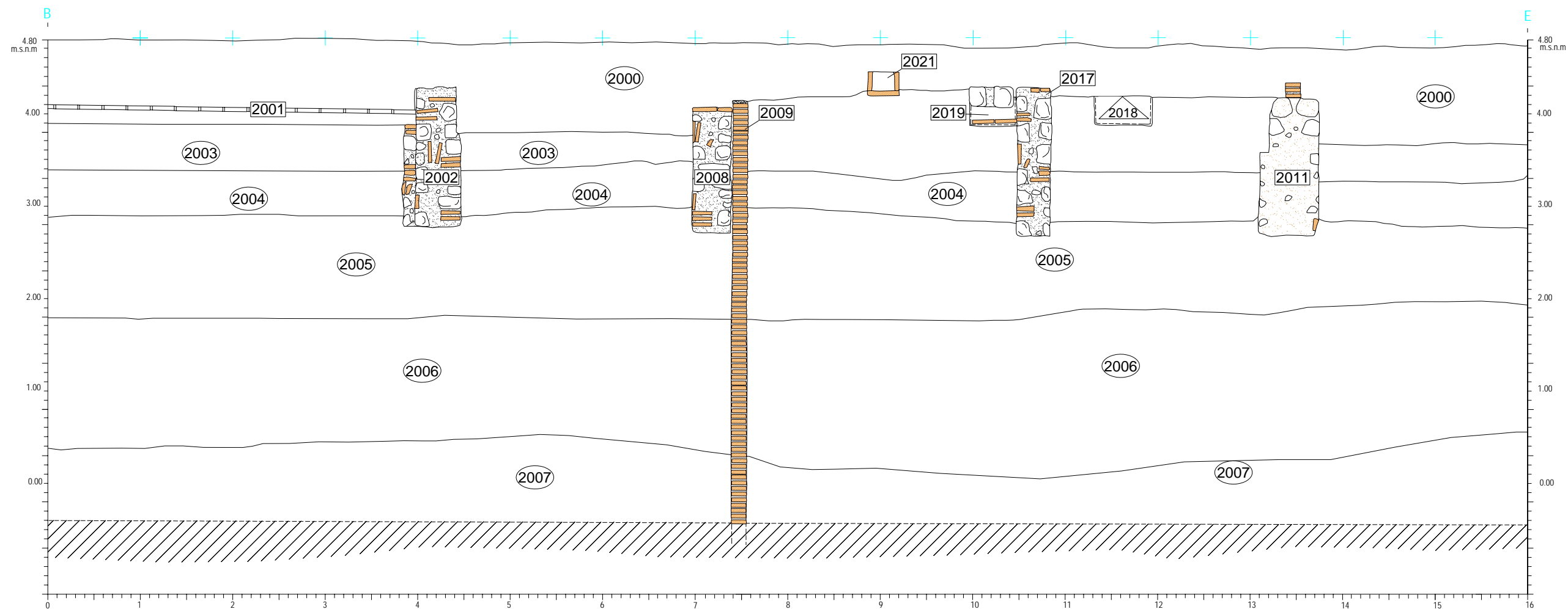
Secció B-B'
